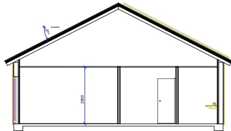
SEKTION A-A
