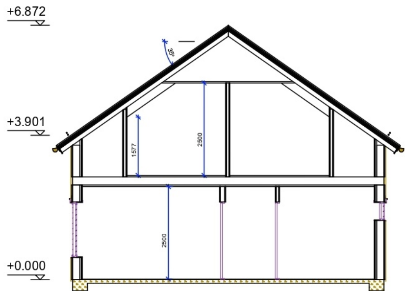
SEKTION A-A
