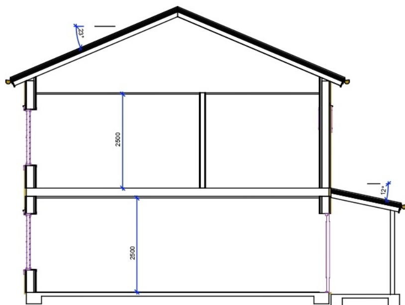
SEKTION A-A
