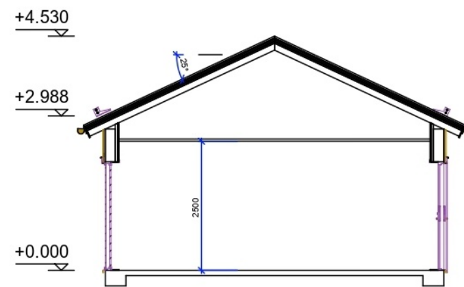
SEKTION B-B
