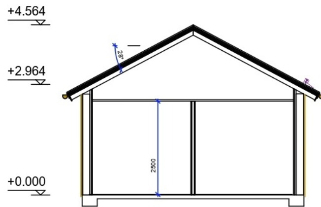
SEKTION A-A
